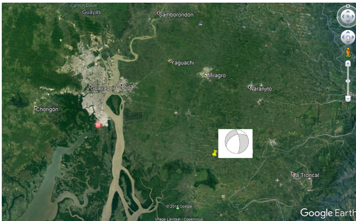
Figura 1. Localización del sismo ocurrido el día de hoy.
