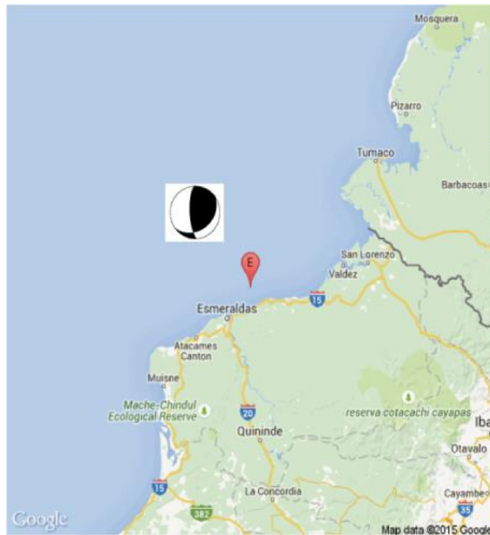
Figura 1. Localización del sismo del 30 de mayo frente a las costas de Esmeraldas. Mecanismo de ruptura principalmente inverso.
